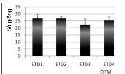
Hình 2. Số giống của tuyến trùng tại các điểm nghiên cứu
