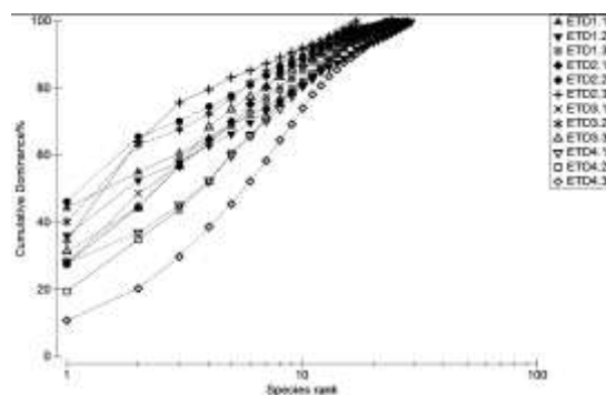
Hình 6. Đường cong K-dominance
