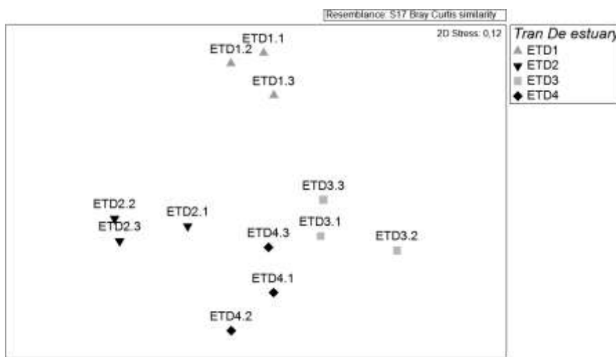
Hình 4. MDS của quần xã Tuyến trùng cửa sông Trần Đề
