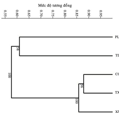
Hình 2: Biểu đồ so sánh mức độ tương đồng về thành phần loài TMCB ở cận ở khu BTTN Tà Xùa với các khu vực lân cận theo tập hợp nhóm giá trị gốc nhánh với 1000 lần nhắc lại; Tên viết tắt các khu vực: TX = Tà Xùa, XN = Xuân Nha, CO = Copia, PL = Pù Luông, TD = Tam Đảo
