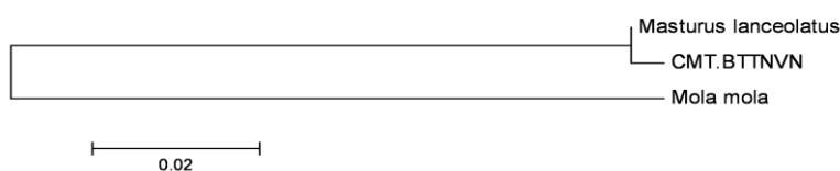
Hình 3: Mối quan hệ họ hàng của loài cá mặt trắng nghiên cứu (CMT_BTTNVN) với loài Masturus lanceolatus (KF930108) và loài Mola mola (JQ775087) đã công bố trên Genbank Mẫu cá mập (CM_BTTNVN)
