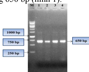
Hình 1: Kết quả điện di sản phẩm PCR các mẫu nghiên cứu trên gel agarose 1,2%
