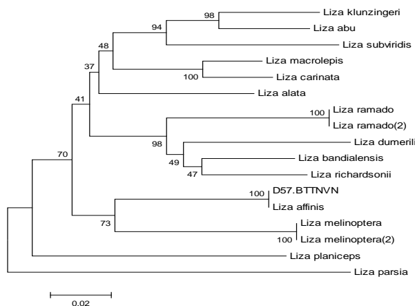
Hình 9: Mối quan hệ họ hàng của loài cá đối vây trước D57_BTTNVN với 14 loài thuộc giống Liza
